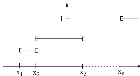
FIG. 3.1 – Exemple de fonction de répartition d'une v.a.r. simple
