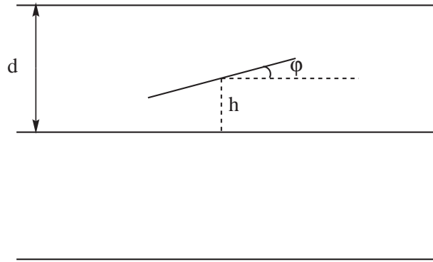
FIG. 3.2 – Aiguille de Buffon
