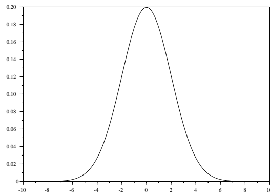
FIG. 1.1 – u_3(x, y) avec x = 2
